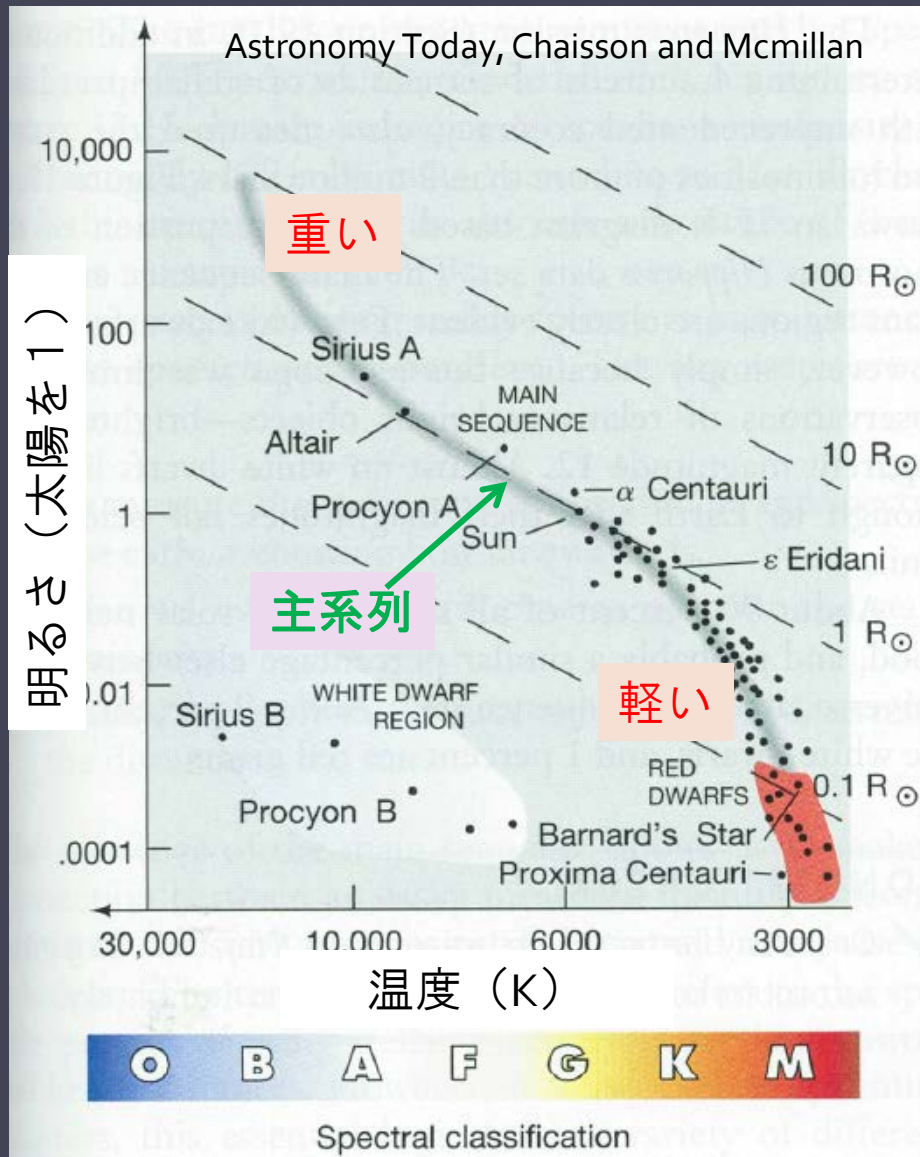
太陽近傍5pcの星のHR図
